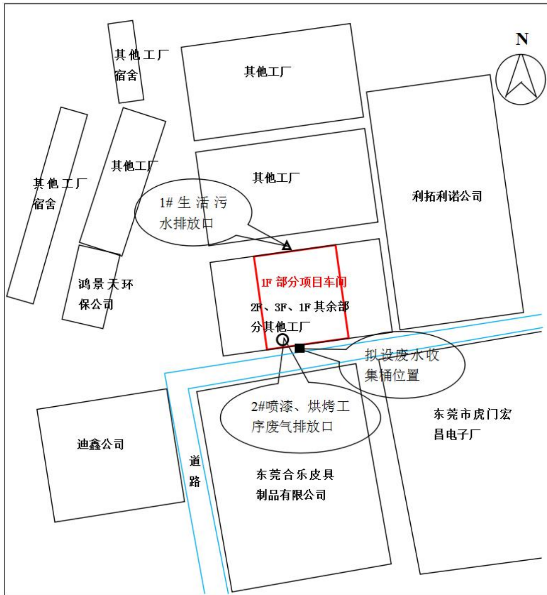
图3-1 厂区平面布置及监测点位
